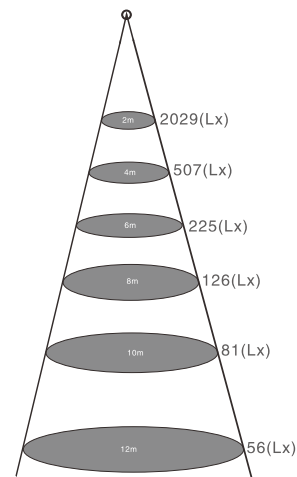
180W路燈 照度分布圖
