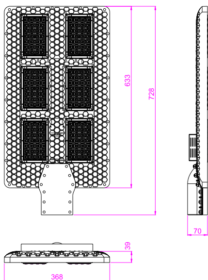
尺寸圖 Size
